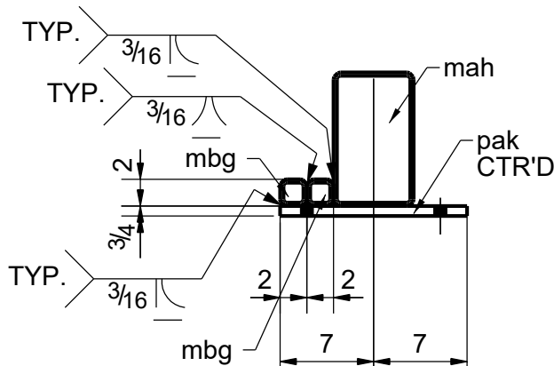
J - J
